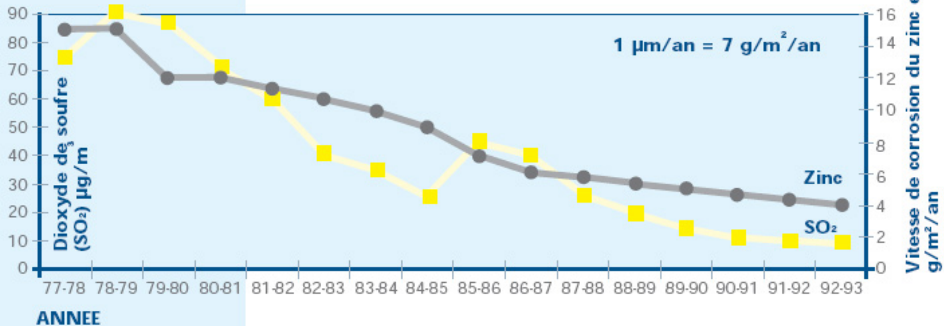
Figure 4 : Niveaux de dioxyde de soufre mesurés à Stockholm, Suède, et vitesse de corrosion du zinc dans cette même ville. Les concentrations en SO 2 indiquées correspondent à des valeurs moyennes pour la période hivernale. Knotkova et Porter, 1994.
